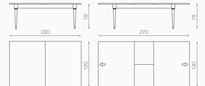
TAVOLO ALLUNGABILE / EXTENSIBLE TABLE 120X220 CM ALLUNGATO / EXTENDED 120X270 CM
