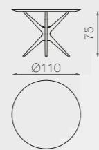
TAVOLO TONDO Ø 110 / ROUND TABLE Ø 110
