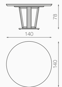
TAVOLO TONDO Ø 140 / ROUND TABLE Ø 140
