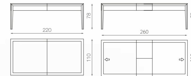
TAVOLO ALLUNGABILE / EXTENSIBLE TABLE 110X220 CM ALLUNGATO / EXTENDED 110X300 CM
